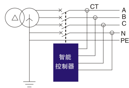
图2 4PT型
