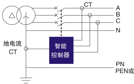
图4 (3P+N)W型
