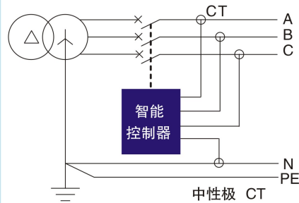
图3 (3P+N)T型
