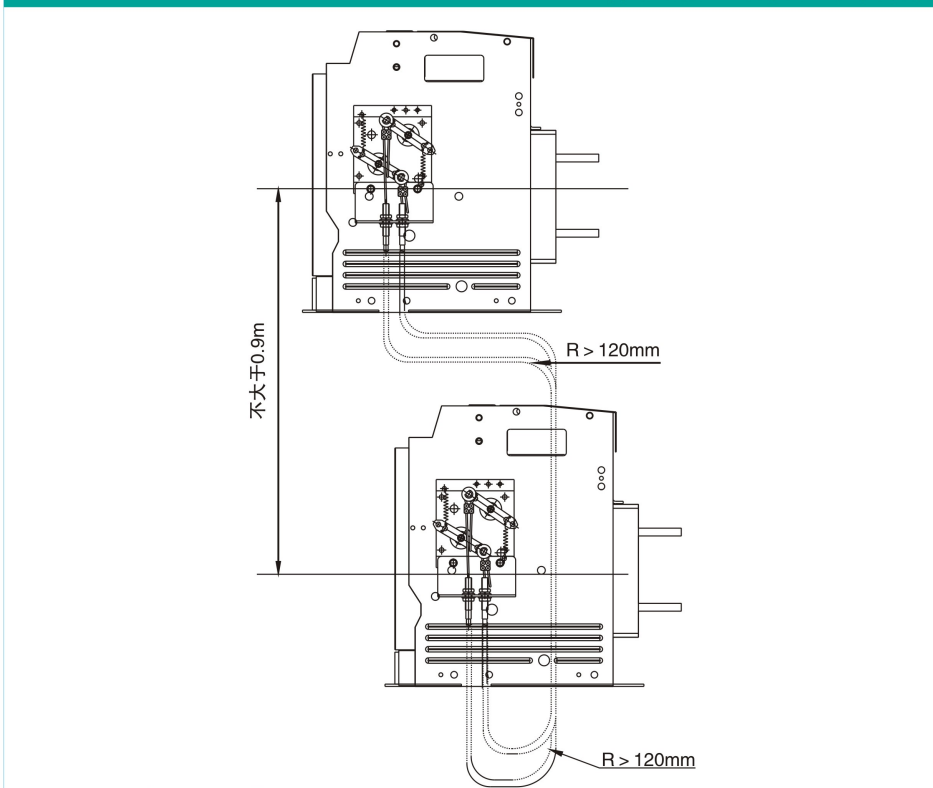
两台断路器之间的垂直机械联锁
